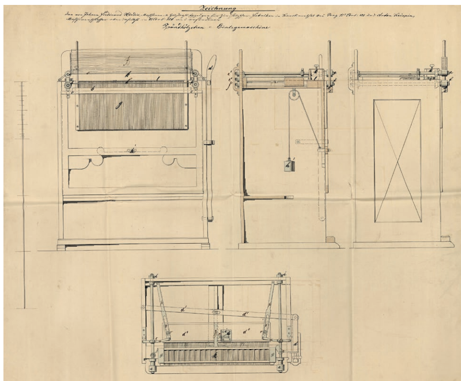
Obr. 3 – Schéma základního stroje – výřez z privilegia No. 4522 z roku 1858. Österreichisches Patentamt, Abteilung Bibliothek und Dokumentation, Wien.
