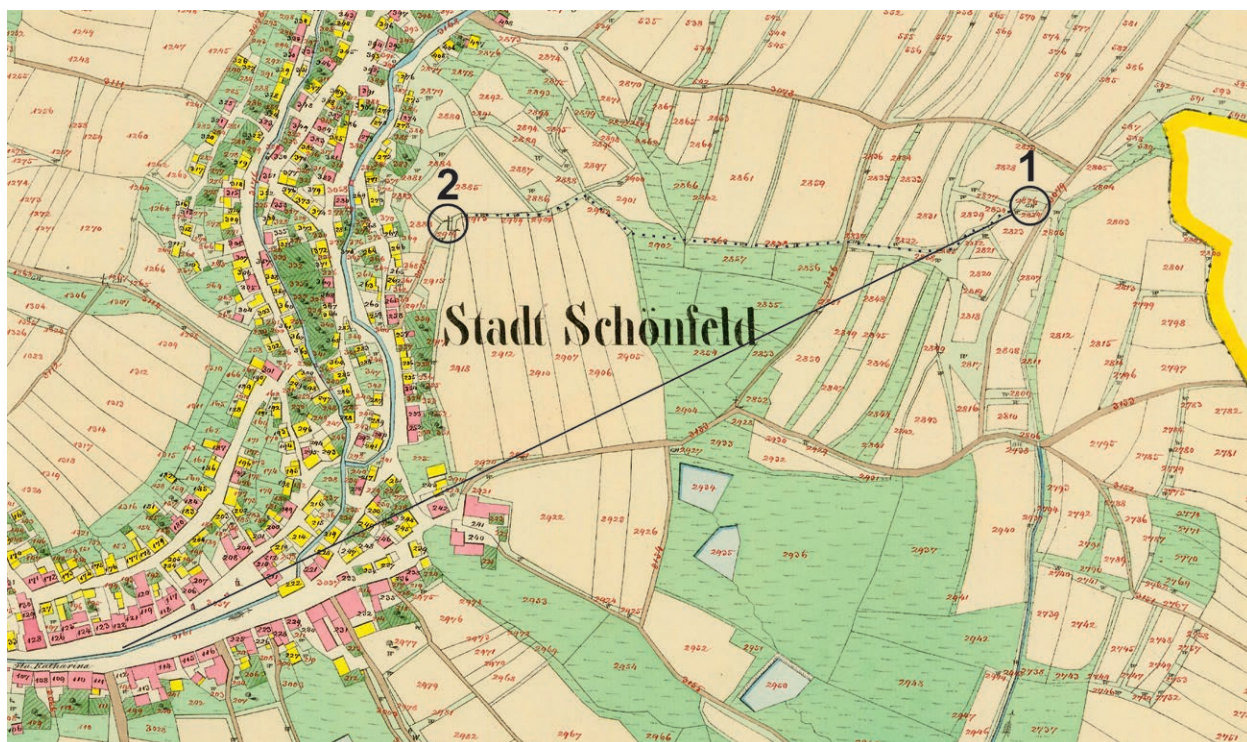
Obr. 12 – Krásno, vyznačení obecní pastviny č. kat. 2826, polohy bývalého popraviště (1), a kříže stojícího na začátku zaniklé cesty (2) vedoucí z města k popravišti (značena tečkovaně). Plnou linkou zvýrazněna pohledová vazba popraviště na hlavní podélnou osu náměstí. ÚAZK, inv. č. 3527; úprava J. Krček.
