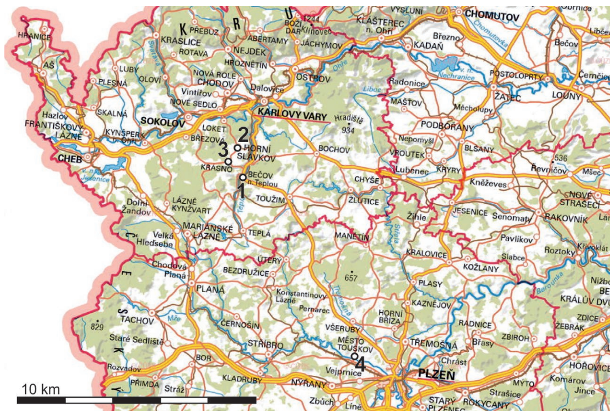
Obr. 1 – Kartografické znázornění zpracovaných lokalit: Bečov nad Teplou (1), Horní Slavkov (2), Krásno (3), Město Touškov (4). Současné mapové podklady, není-li uvedeno jinak, https://geoportal.gov.cz/web/guest/map ; úpravy J. Krček.
