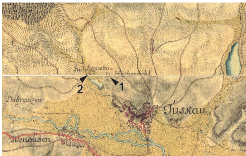
Obr. 14 – Město Touškov, vyznačení polohy šibenice (1) a židovského hřbitova (2) na prvním vojenském mapování, spojené sekce č. 138 a 156.
